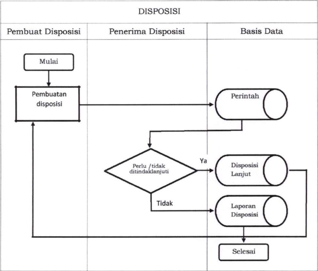
Gambar 4 Alur Disposisi
