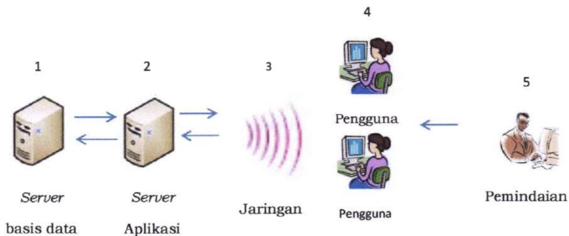
Gambar 1: Arsitektur TNDE
